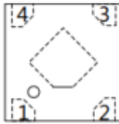
正面透视图
